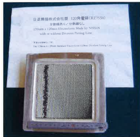
120mm×120mm标准电铸 (照片是无分型线的产品)
